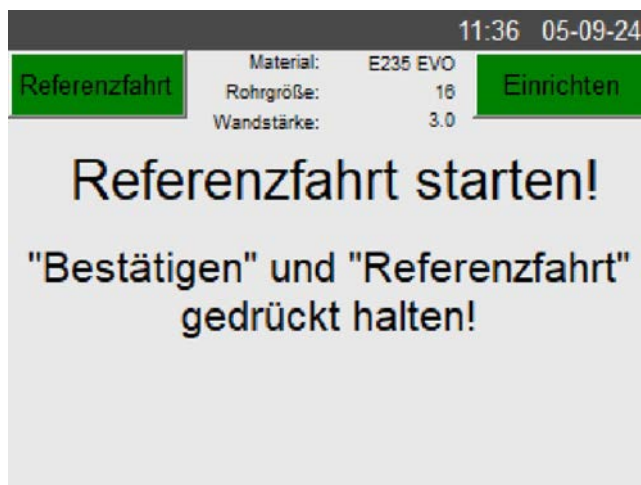
Abb. 55: Referenzfahrt starten
