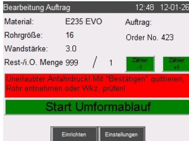
Abb. 80: Unerlaubter Anfahrdruck
