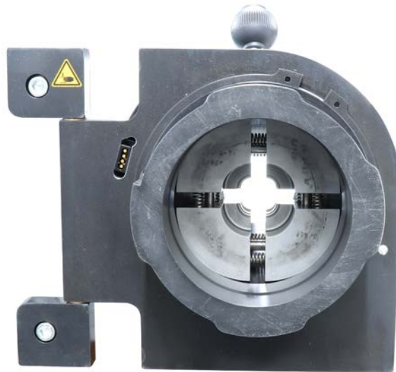
Abb. 52: Formbacken eingesetzt
