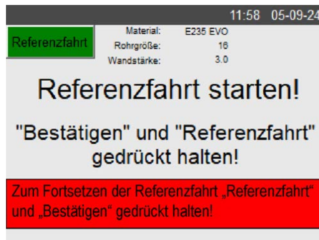
Abb. 17: Referenzfahrt starten
