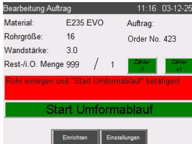
Abb. 19: Start Umformablauf
