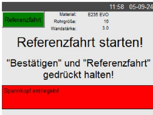
Abb. 13: Spannkopf entriegeln
