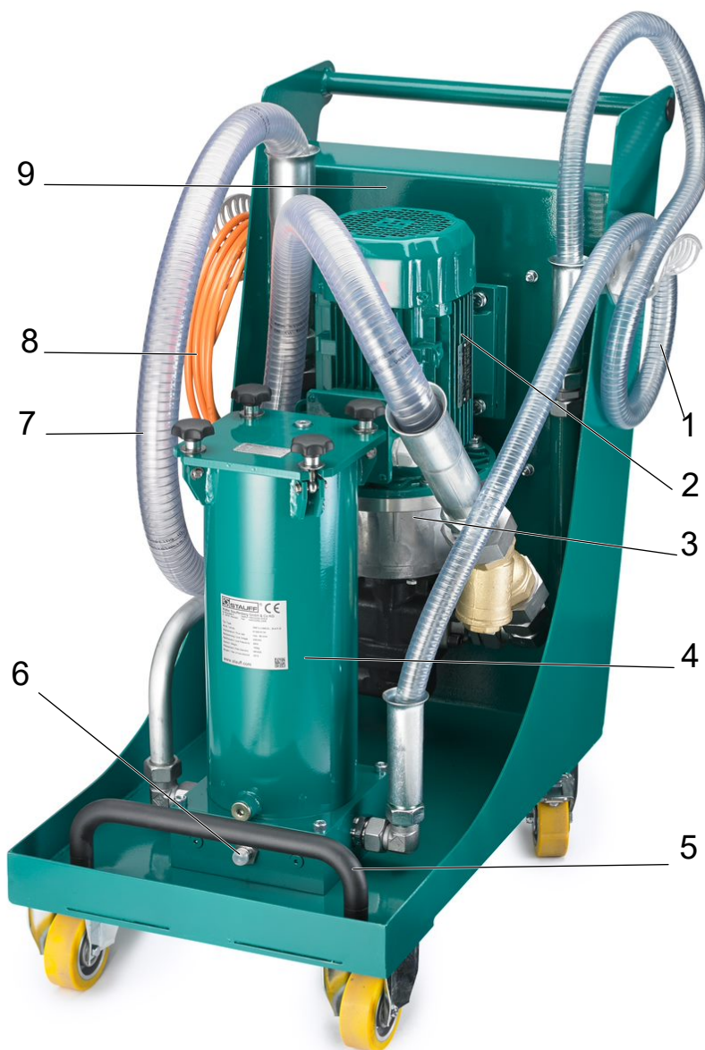
Ilustr. 1: Widok urządzenia
