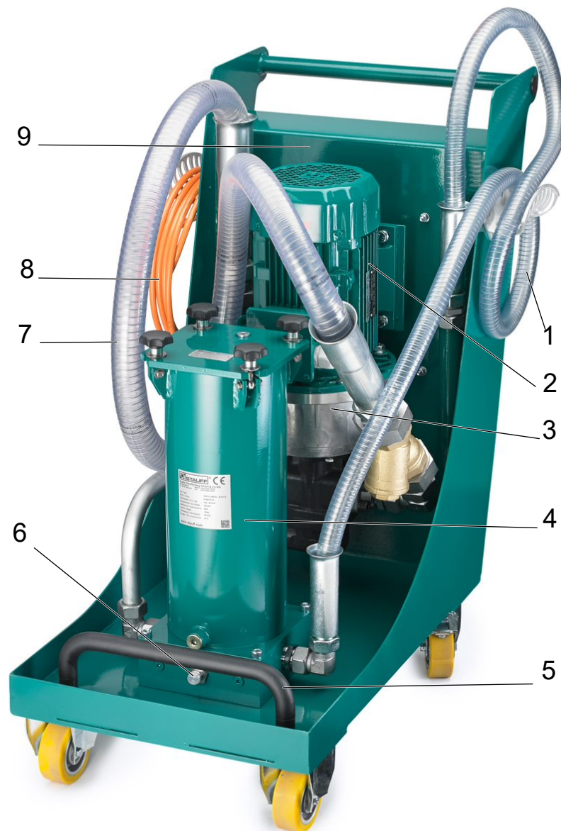
Abb. 1: Gesamtansicht
